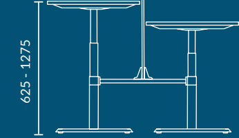
Lano-E 300 T
