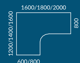
shaped desk Schreibtisch in L-Form Lano-E 300 T
