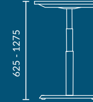
Lano-E 300 T
