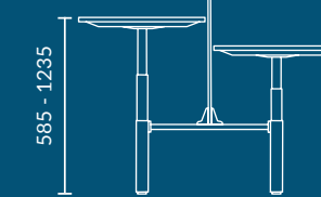
Lano-E 300 F
